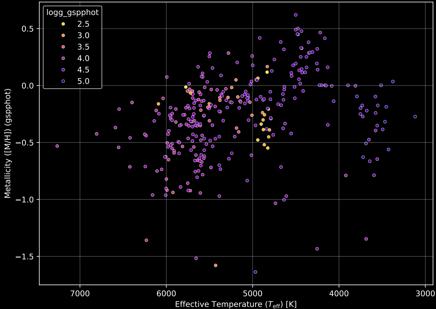
APOGEE DR17 Field: [sgr_tidal10] Stellar Population Parameters (n= 315)
